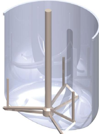
Якорная мешалка петлевого типа
