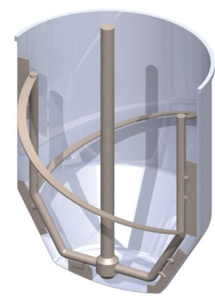
Ленточная якорная мешалка петлевого типа
