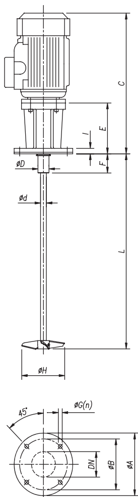
Røreværksflange
