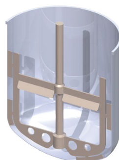
Вариант 03: U-образная якорная мешалка с лопастью
