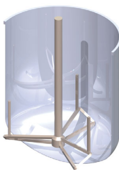
Вариант 05: Якорная мешалка петлевого типа
