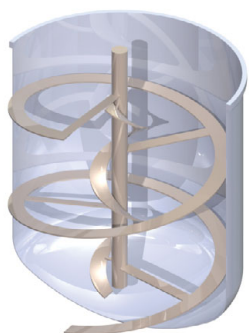
Вариант 04: Ленточная якорная мешалка
