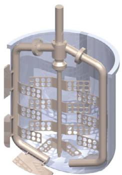
Якорная мешалка с центральным валом с противоположным вращением
