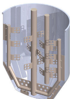
Вариант 02: Якорная мешалка с радиальным отражателем потока
