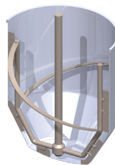
Вариант 06: Ленточная якорная мешалка петлевого типа
