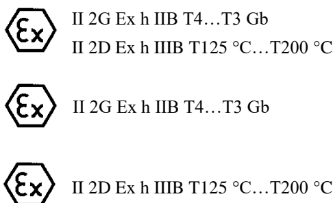
Figure 1.1 : marquage CE ATEX inscrit sur la plaque du fabricant.
